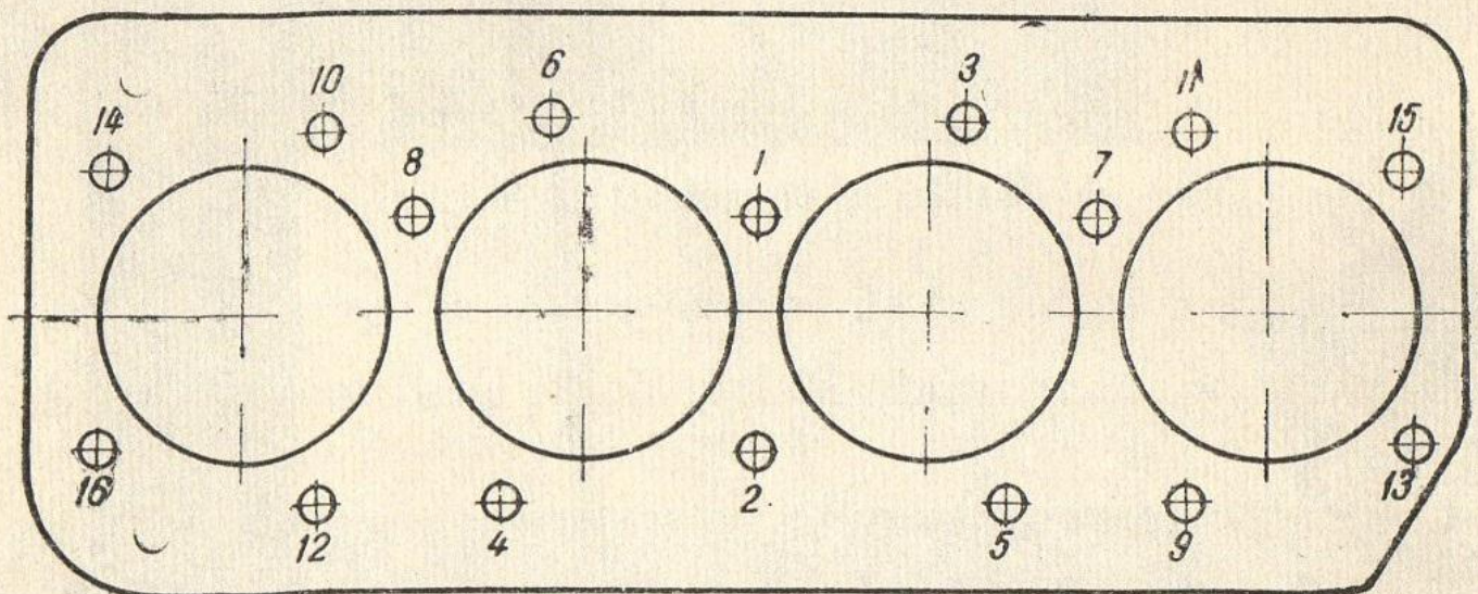
Fig. 39. Ordre de serrage des goujons de culasse
