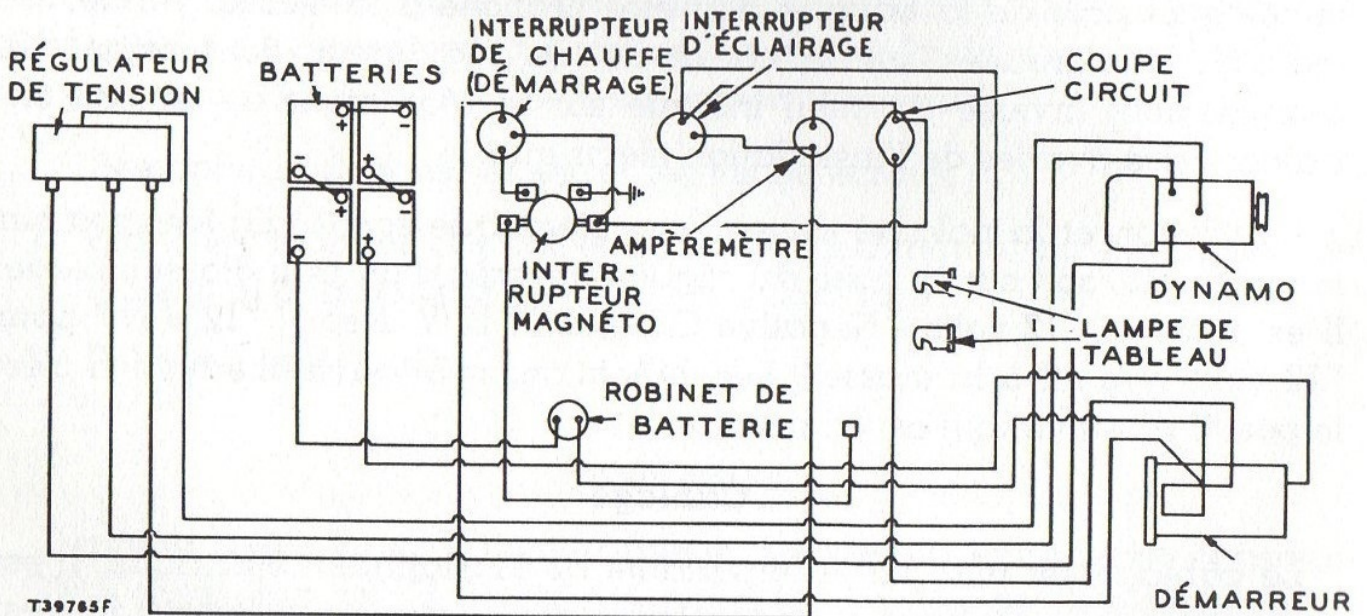
Schéma de câblage — (Démarreur électrique direct) 24 volts
