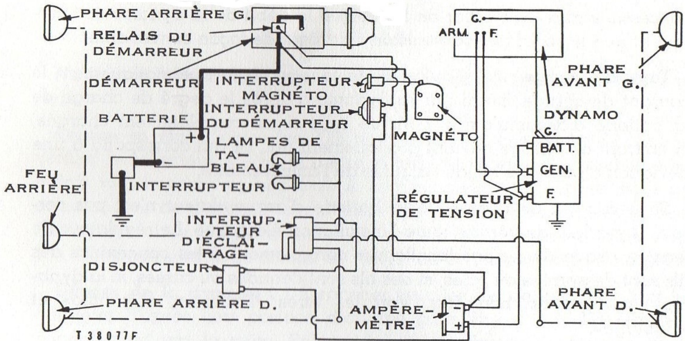
Schéma de l'installation électrique 12 volts
