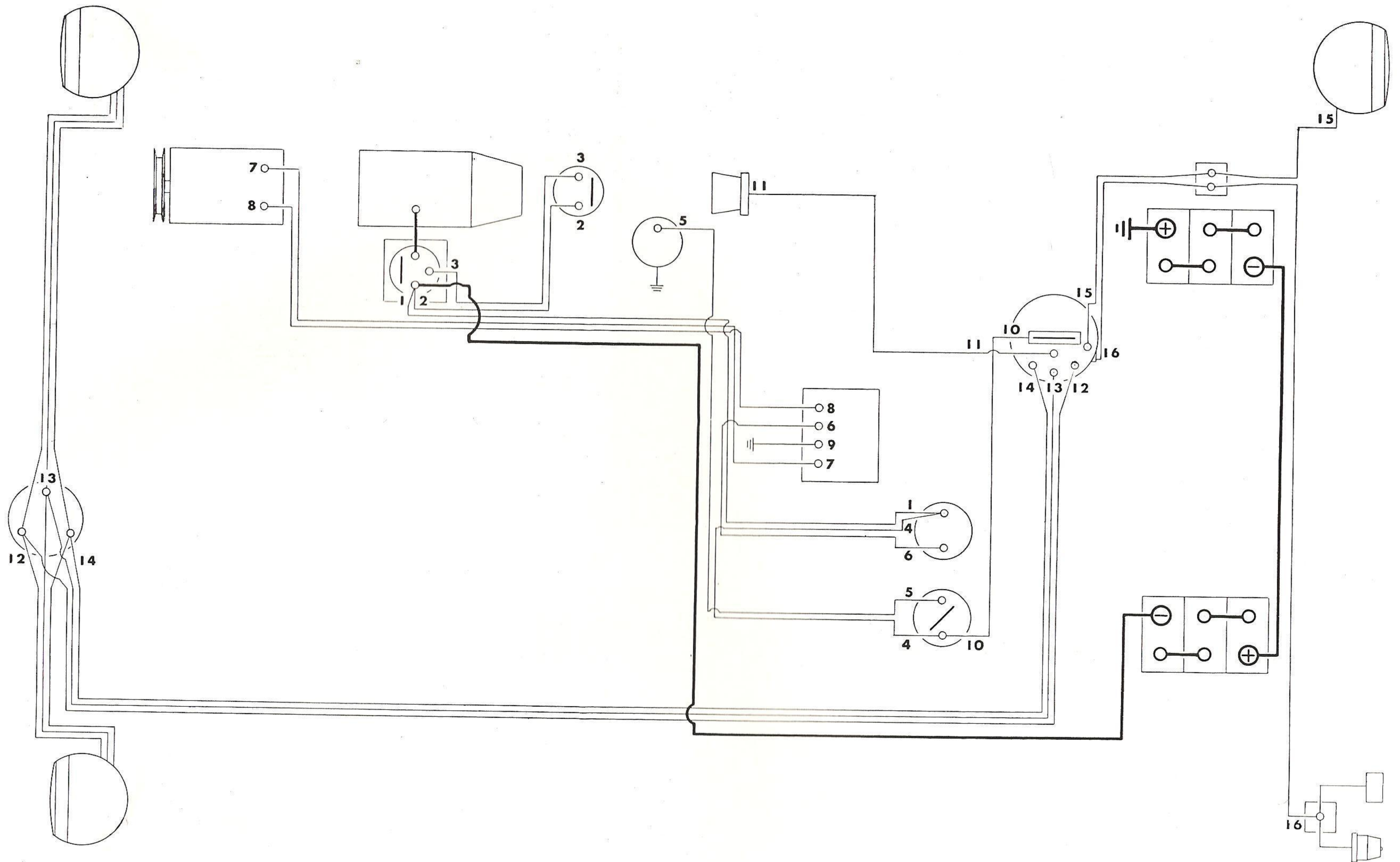
SCHÉMA DE L'ÉQUIPEMENT ÉLECTRIQUE SUR TRACTEUR T.E.F.
