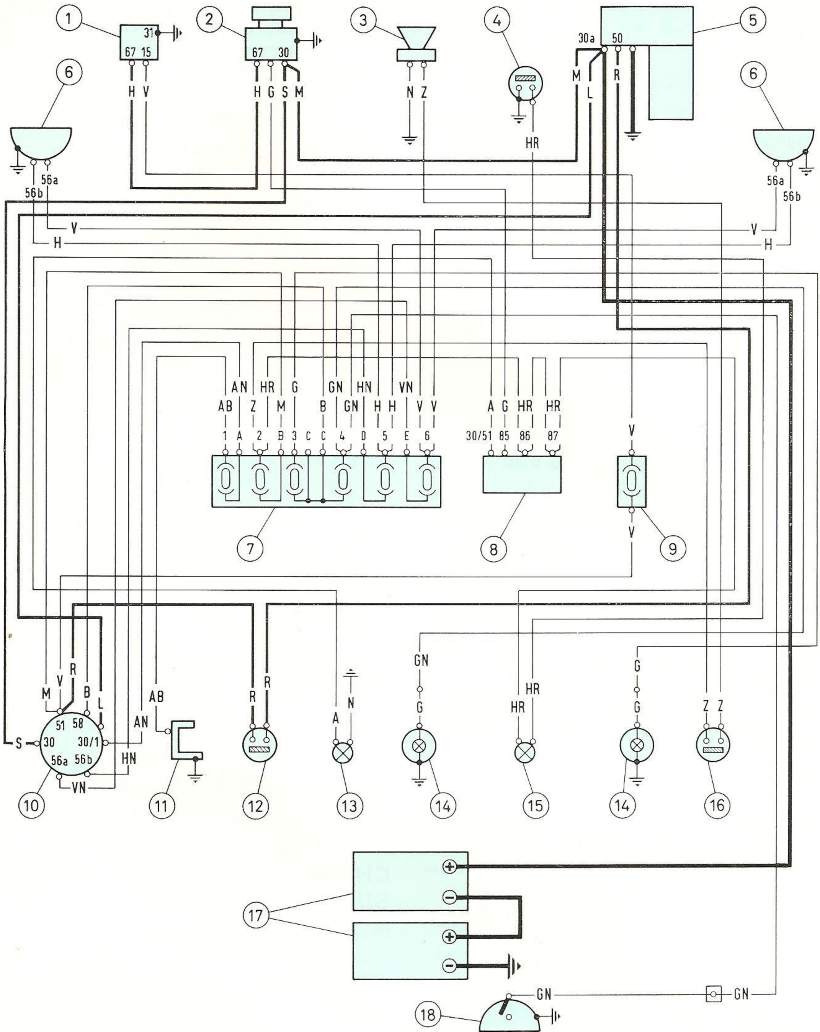
Fig. 27. - Plan de câblage électrique (tension 24 V).
