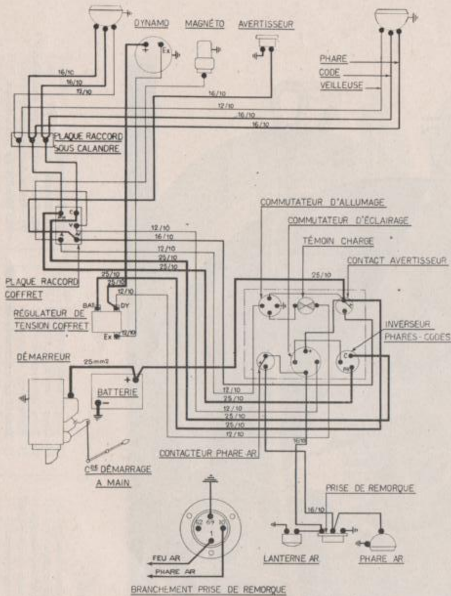
Figure 24. — Schéma de l'installation électrique pour allumage par magnéto.
