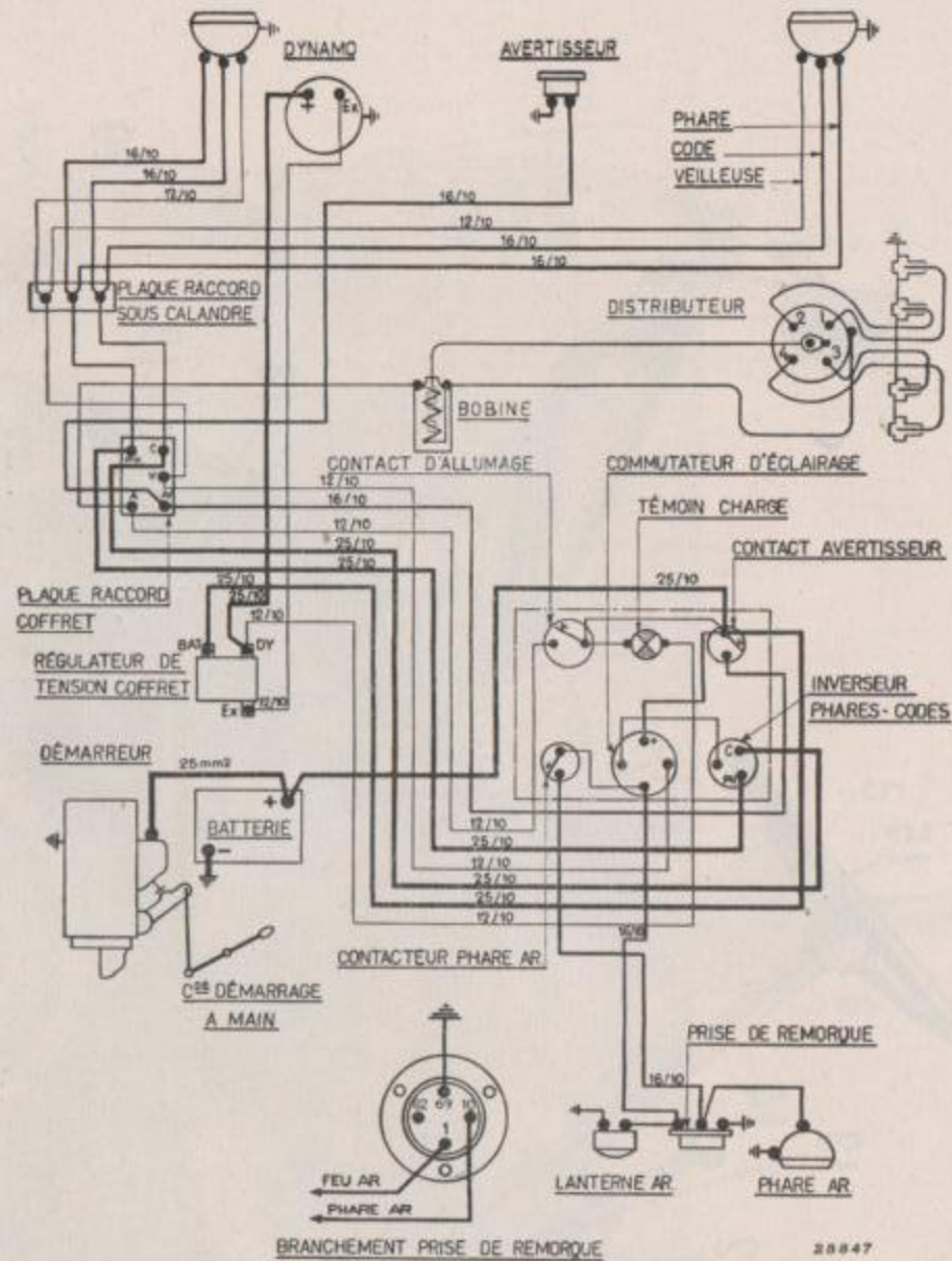
Figure 25. — Schéma de l'installation électrique pour allumage par batterie.
