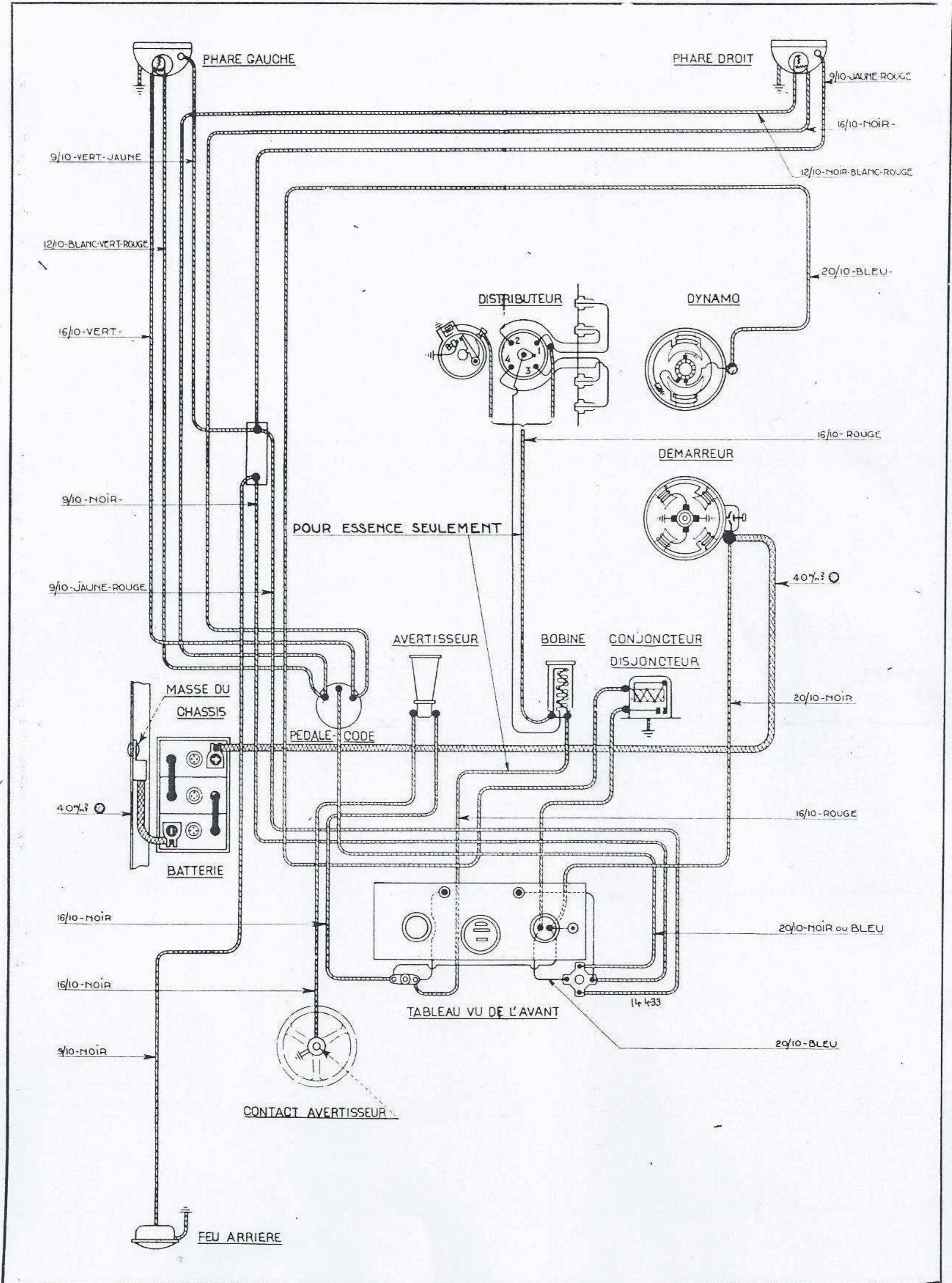
Planche 68. — SCHÉMA D'INSTALLATION ÉLECTRIQUE POUR OSB-PRB-SXB-YFAB-YGAB-YGDB.
