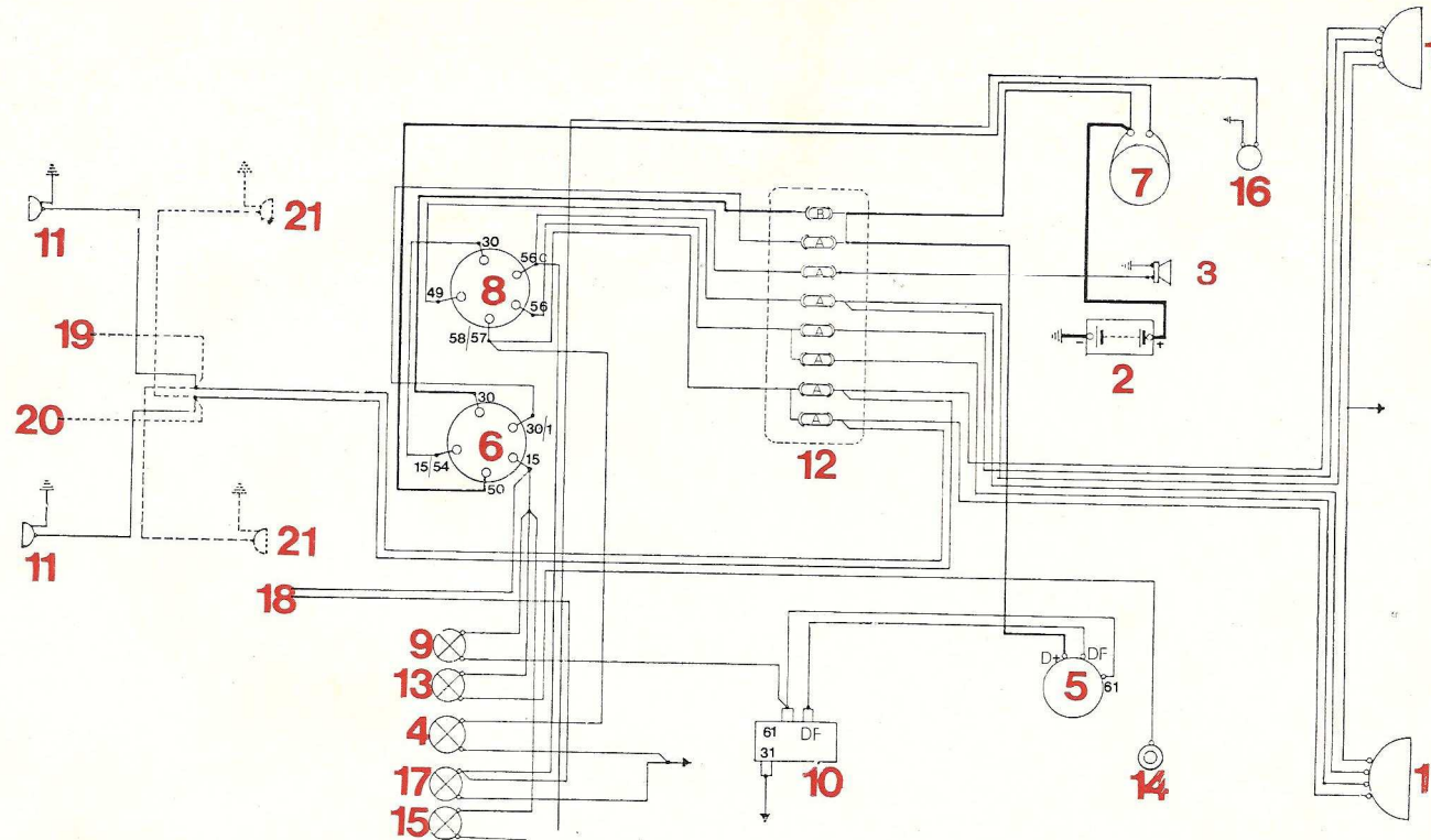
fig. 25 - Schéma de l'installation électrique
