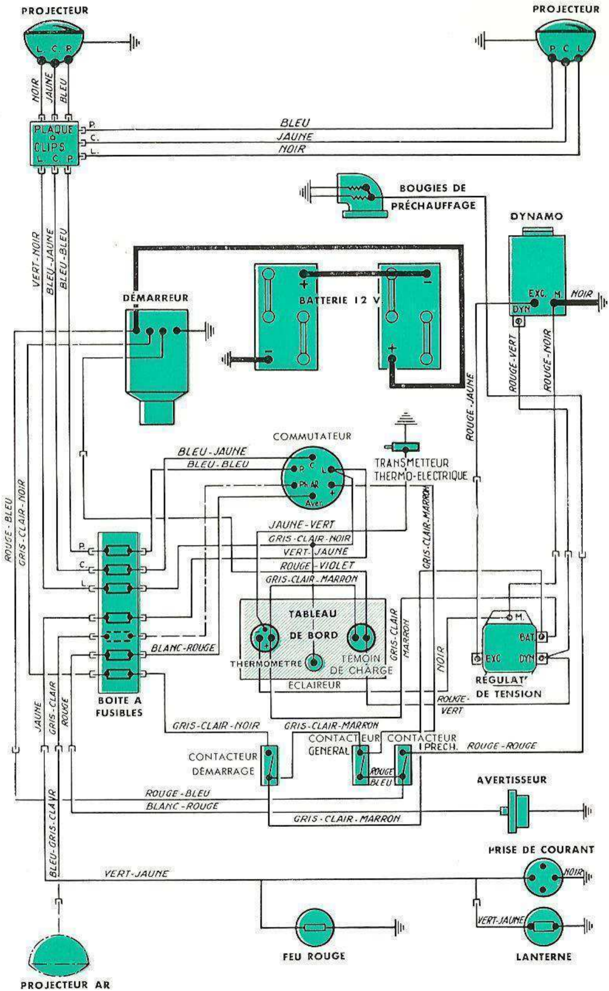
SCHEMA DE L'INSTALLATION ÉLECTRIQUE
