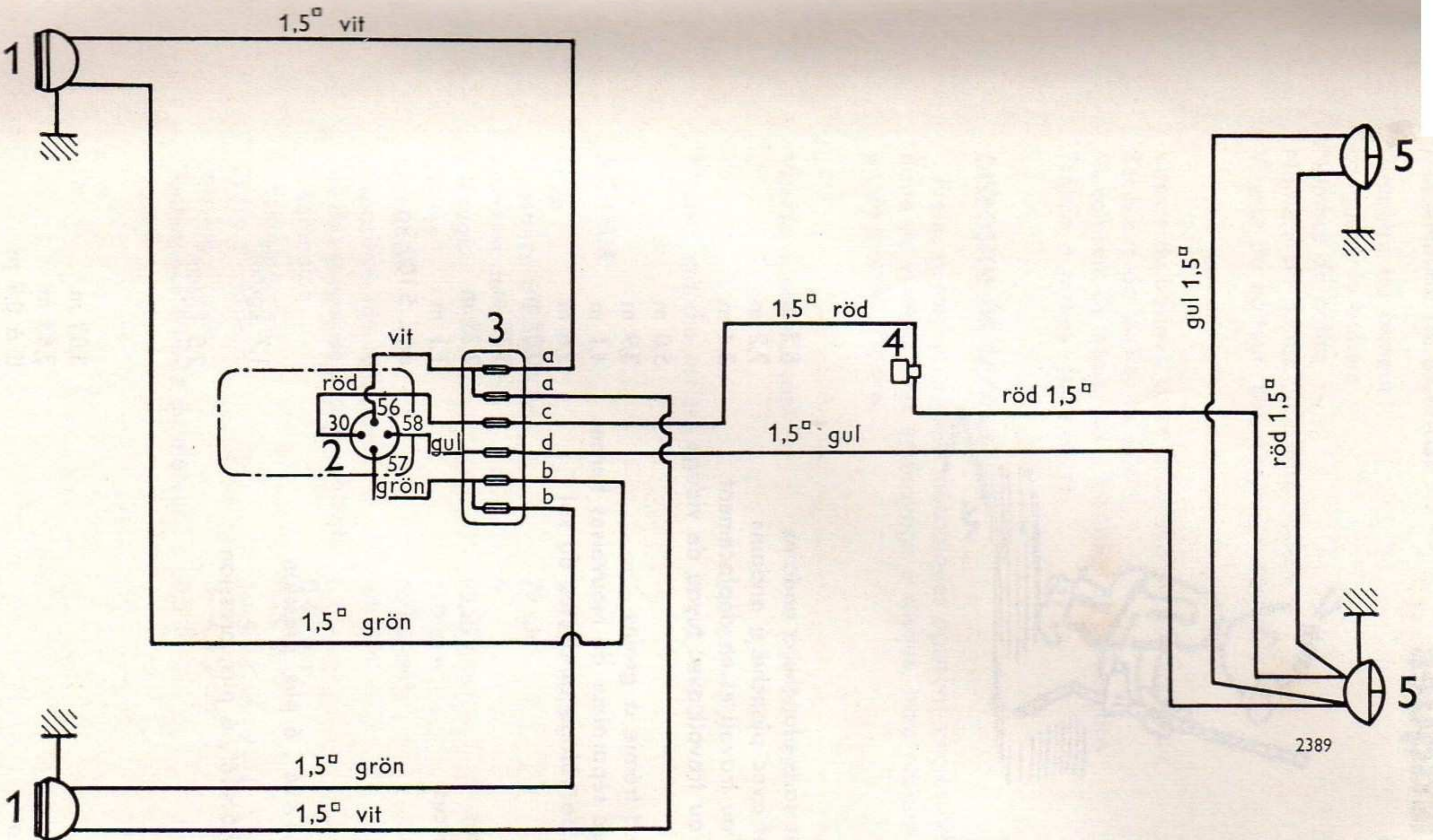
Fig. 56. Schéma de l'installation d'éclairage.
