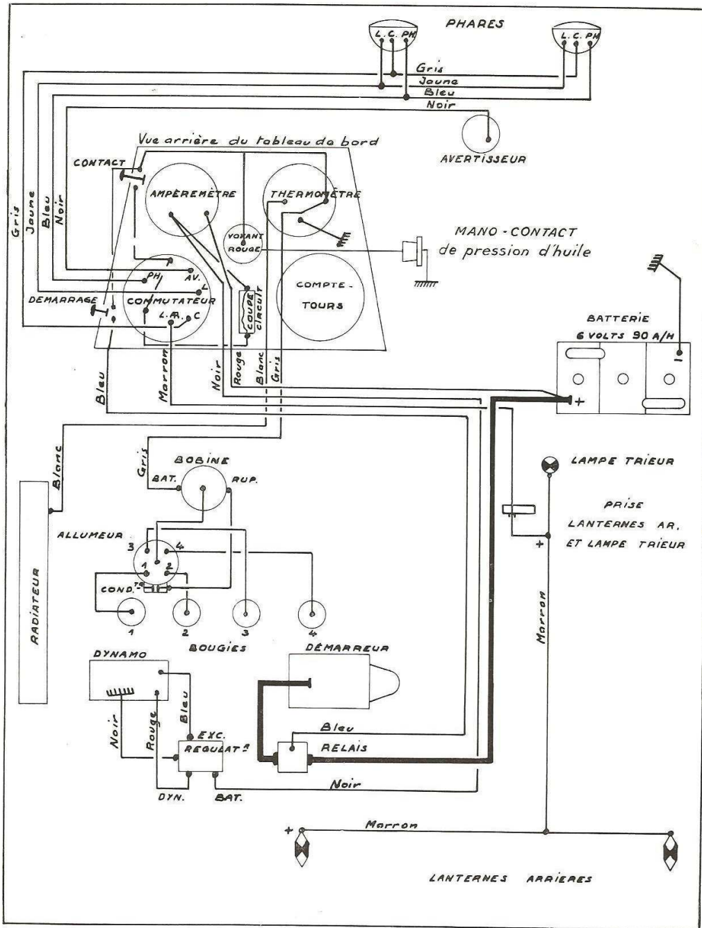
Schéma de l'installation électrique (moteur essence)
