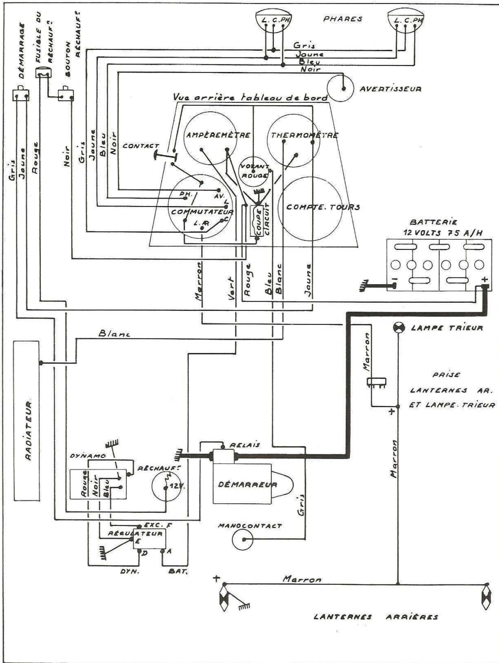
Schéma de l'installation électrique (moteur diesel)
