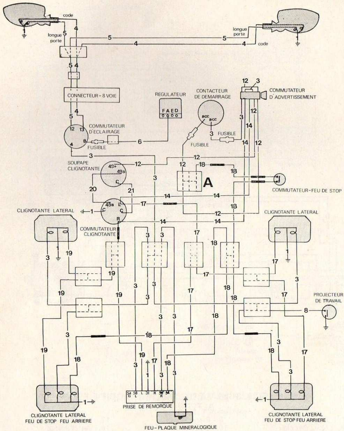
FIGURE 5/32. SCHEMA DE CABLAGE D'ECLAIRAGE A. Connecteur auxiliaire
