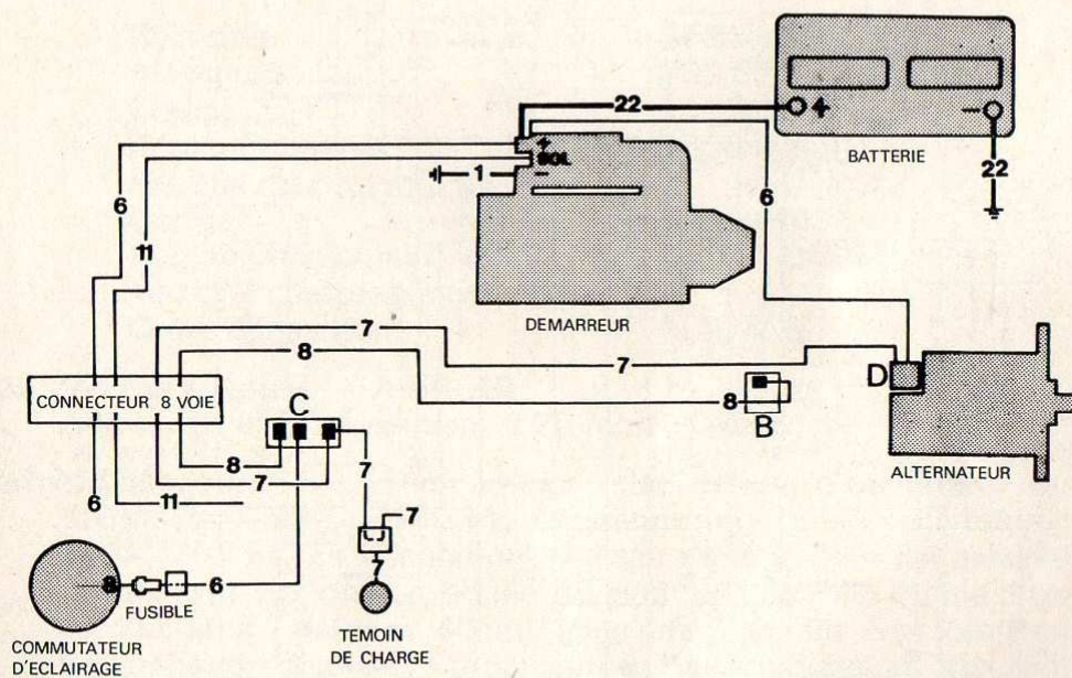
FIGURE 5/31. SCHEMA DE CABLAGE MODIFIE POUR ALTERNATEUR
