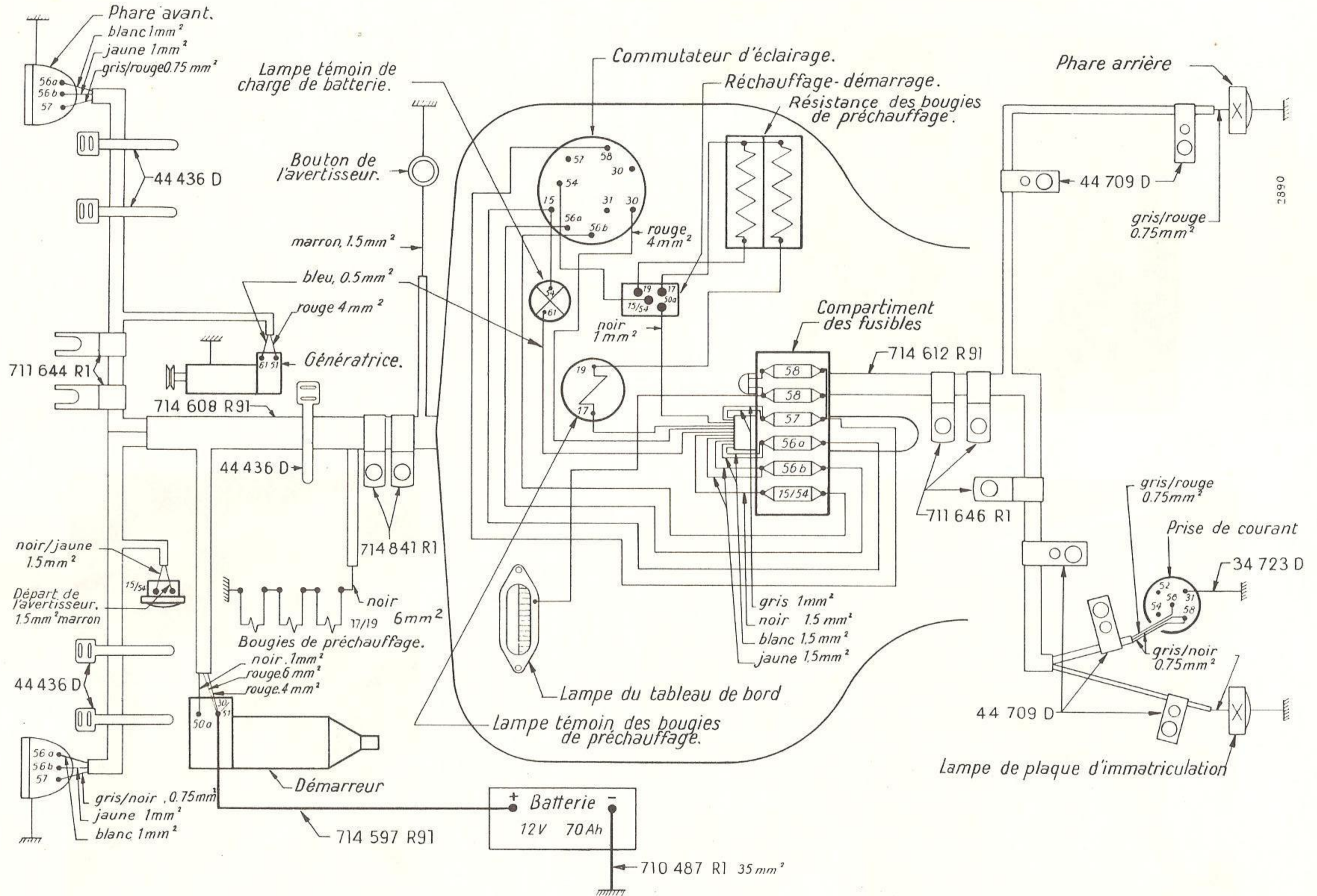
Schéma de câblage
