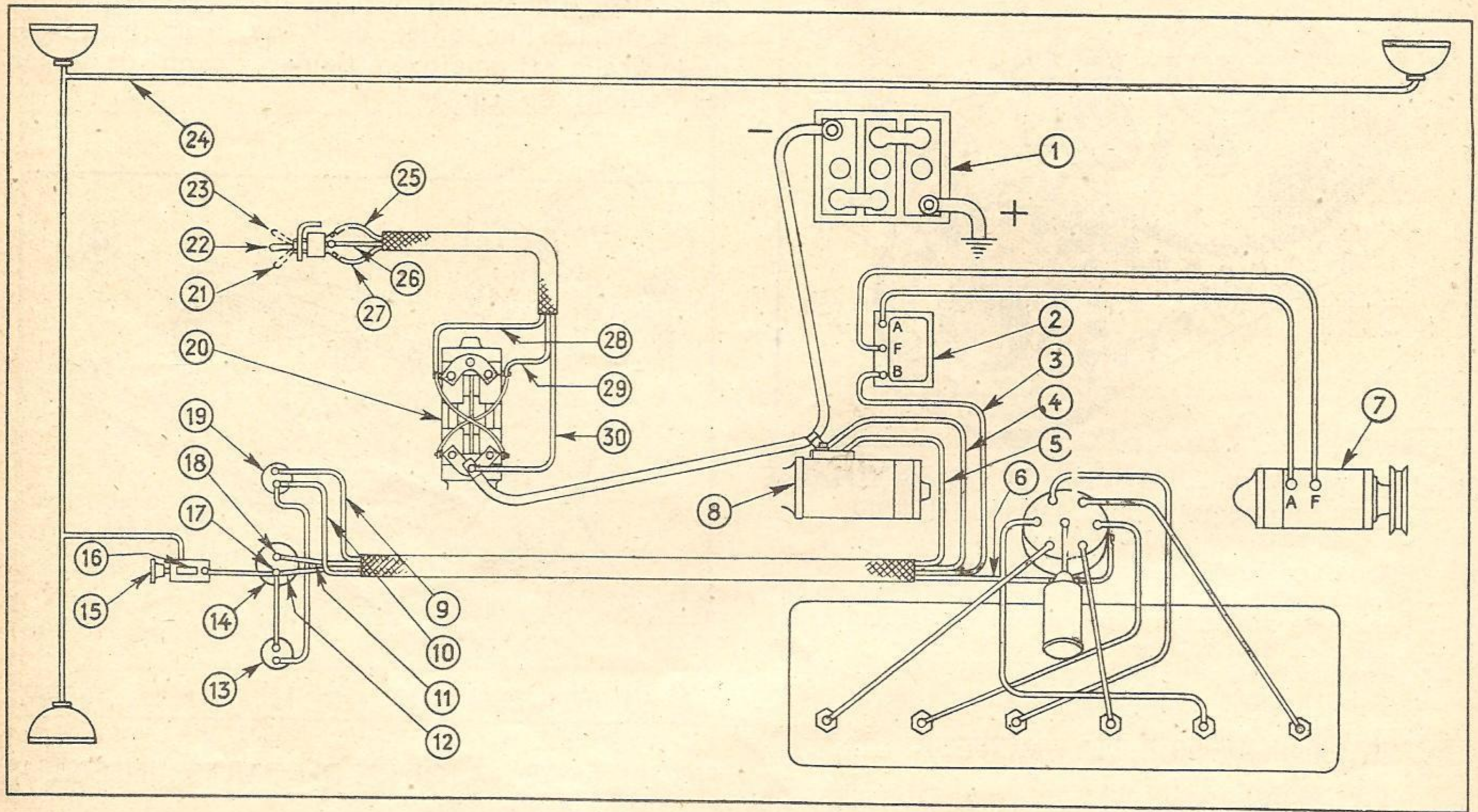
SCHÉMA DU CABLAGE ÉLECTRIQUE
