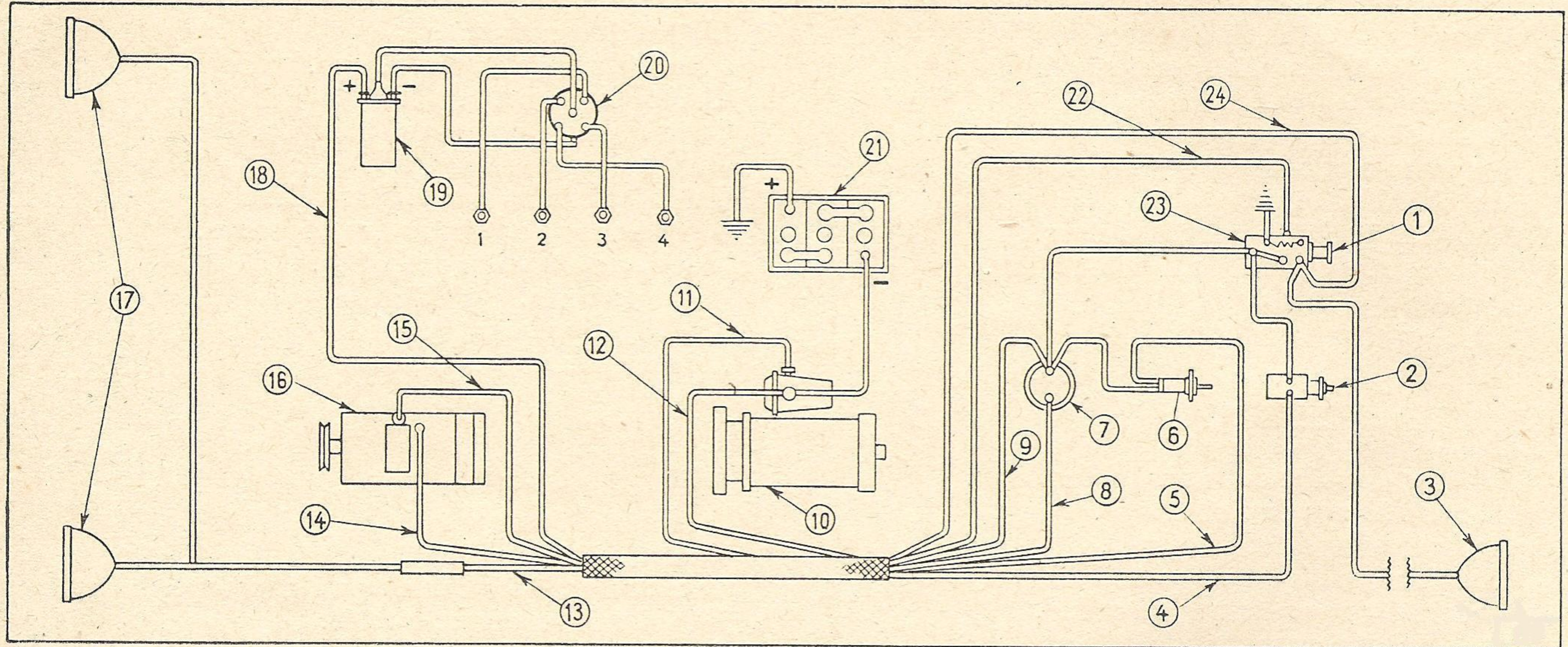
SCHÉMA DU CABLAGE ÉLECTRIQUE.
