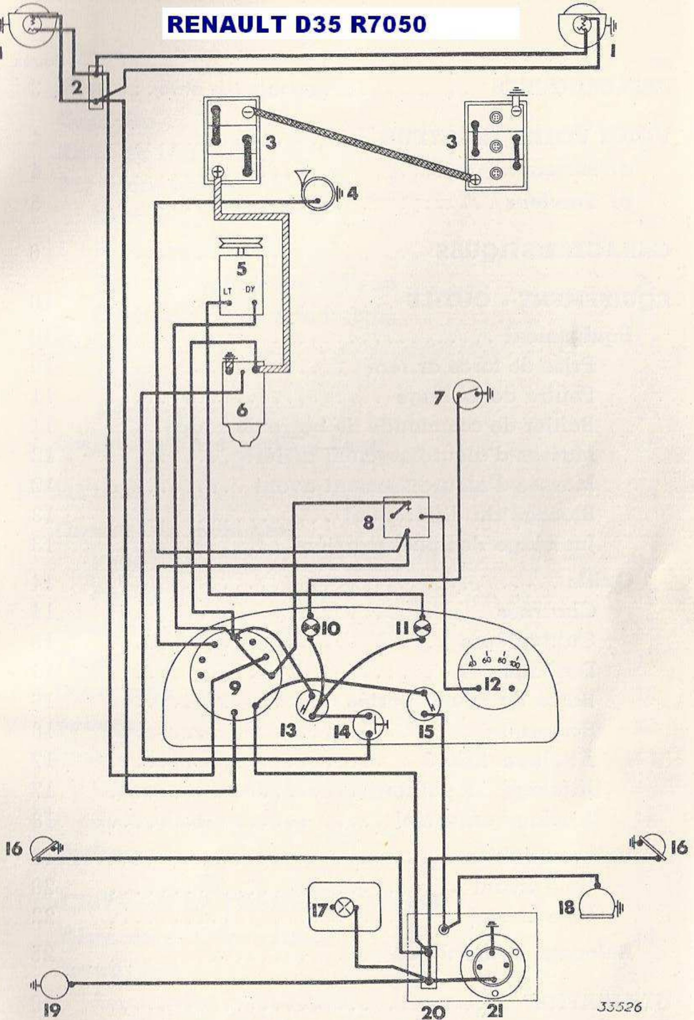
Figure 48. — Schéma d'installation électrique.
